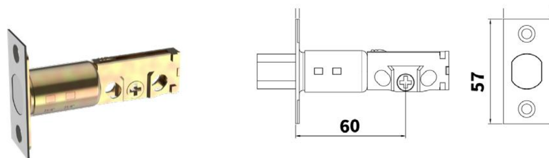
DEADBOLT LTACH
