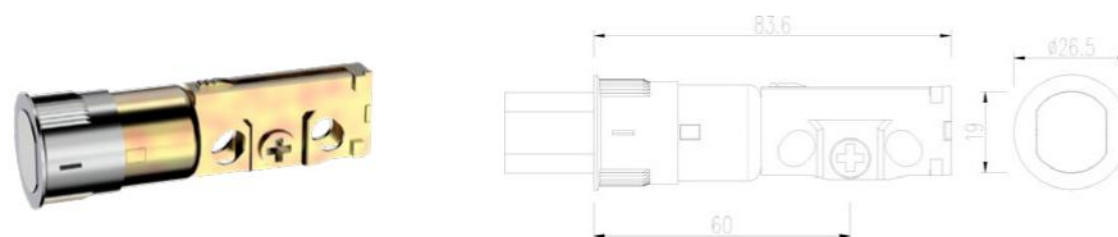
ROUND DEADBOLT LTACH
